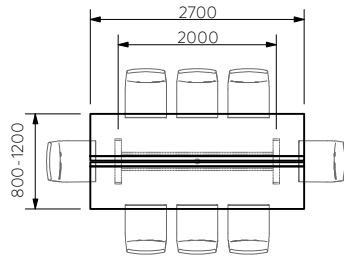
CABLE TRAY 2000/1920
